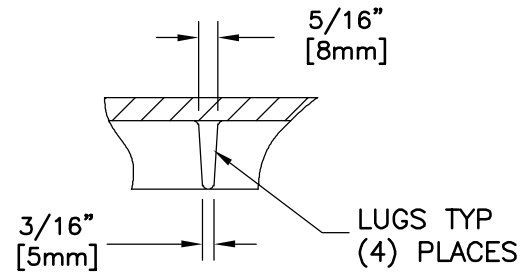
LUG DETAIL TYP (4) PLACES
